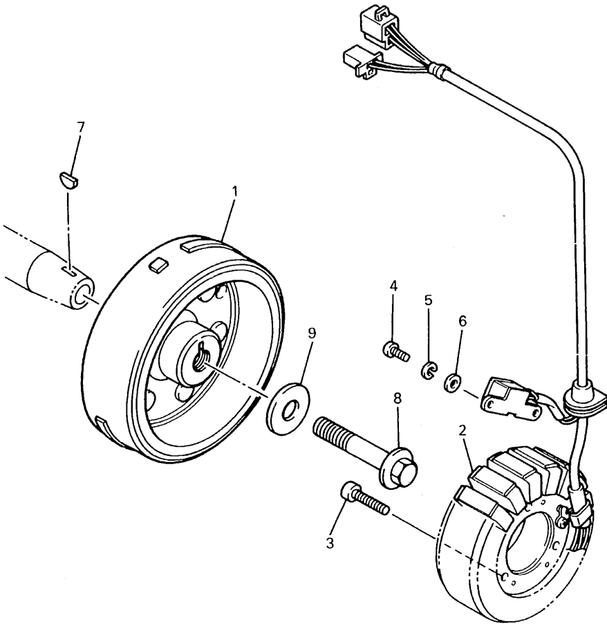
FIG. 39 GENERADOR
