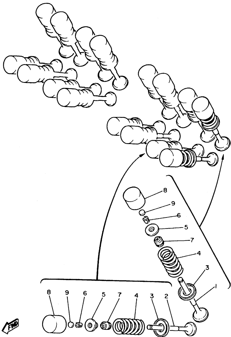
FIG. 4 VALVULA
