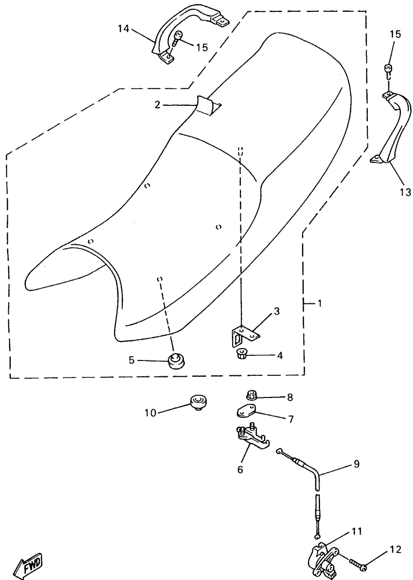
FIG. 28 ASIENTO
