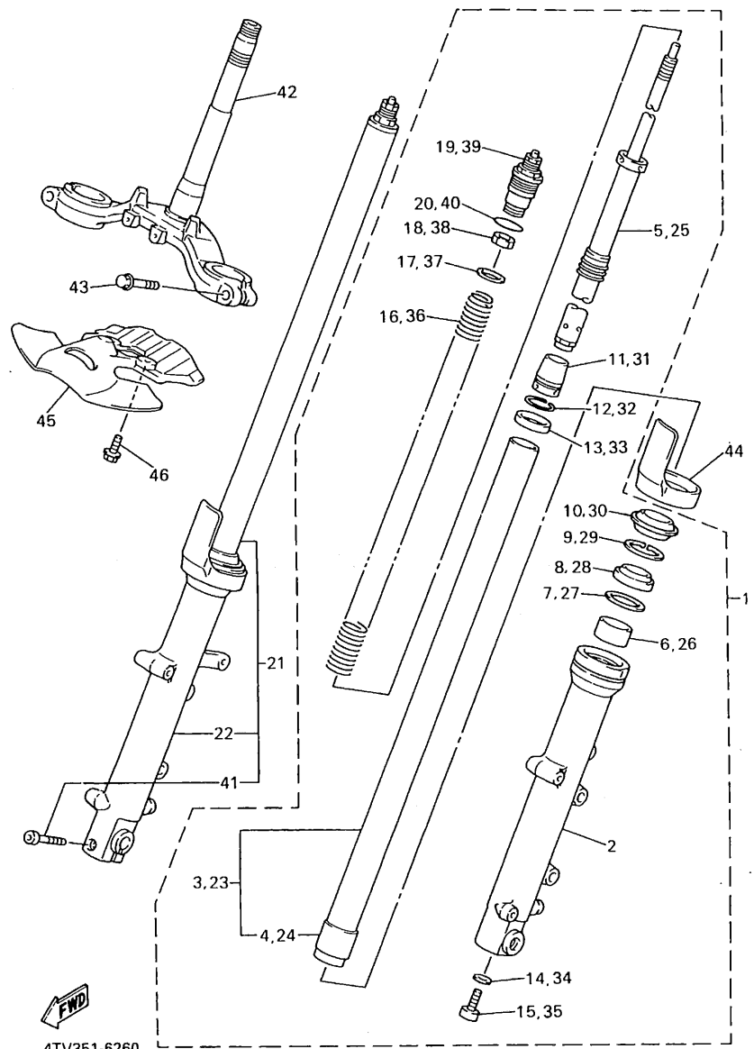
FIG. 26 HORQUILLA DELANTERA
