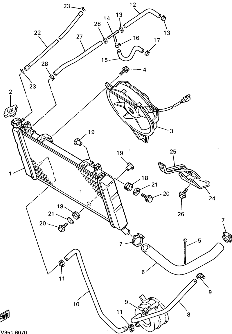
FIG. 7 RADIADOR. MANGUELA
