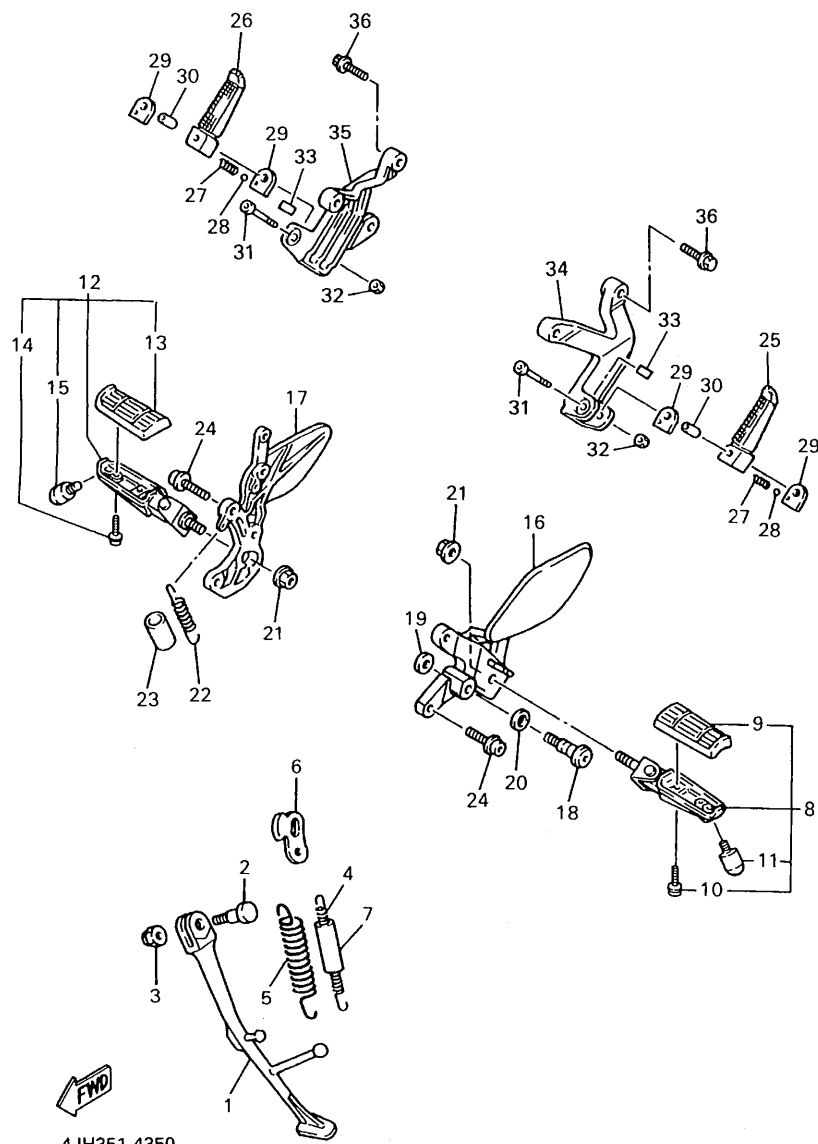
FIG. 35 SOPORTE. APOYAPIE
