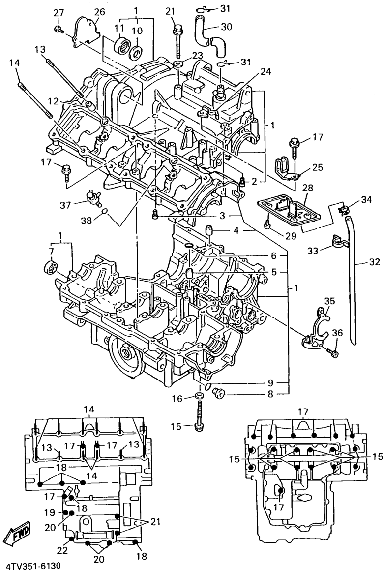
FIG. 13 CARTER
