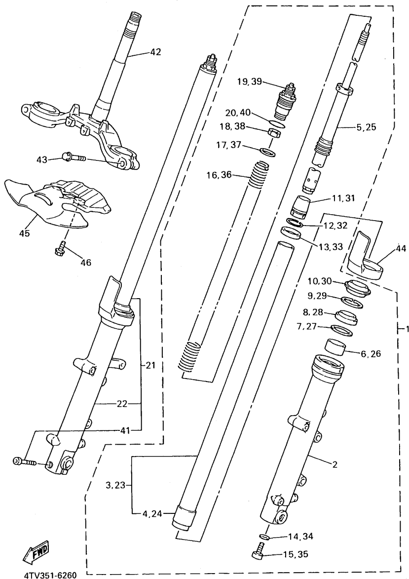
FIG. 26 HORQUILLA DELANTERA
