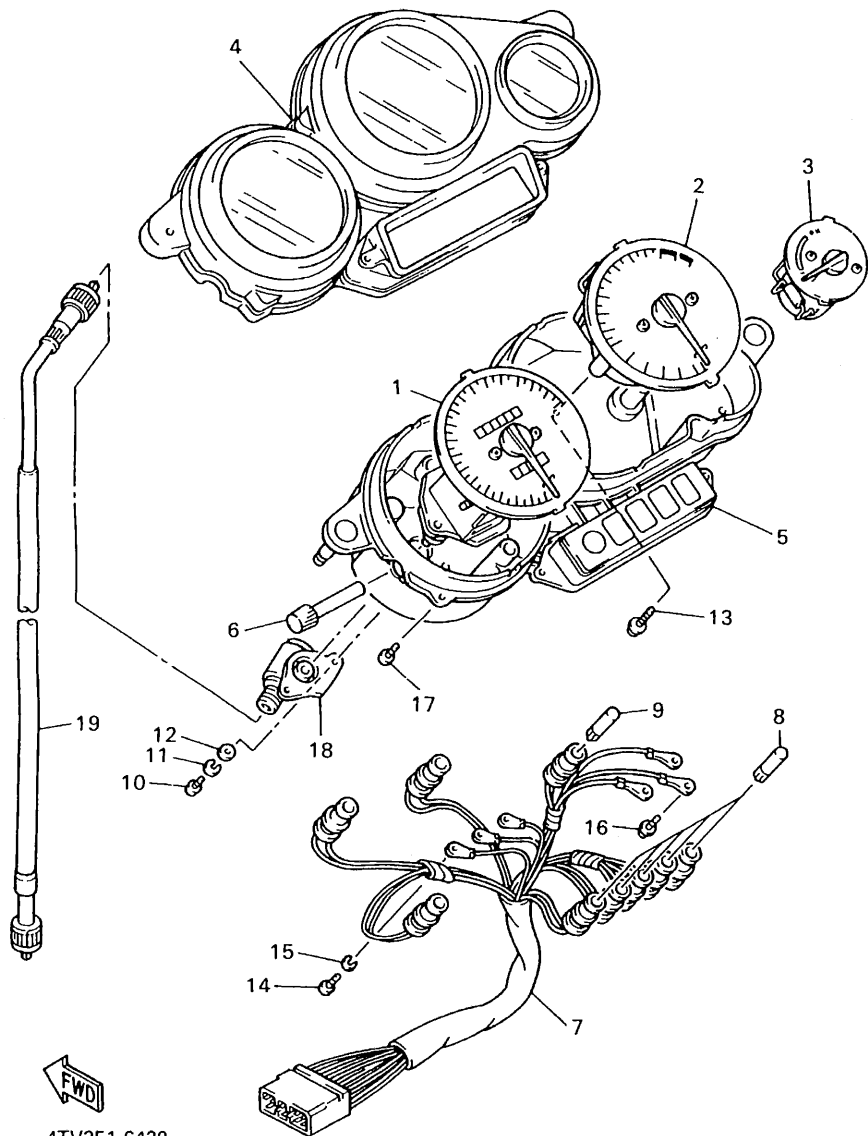
FIG. 42 MEDIDOR
