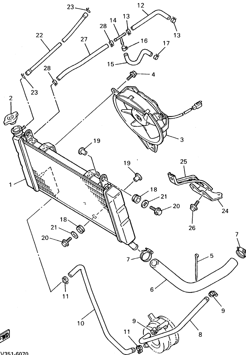
FIG. 7 RADIADOR. MANGUELA
