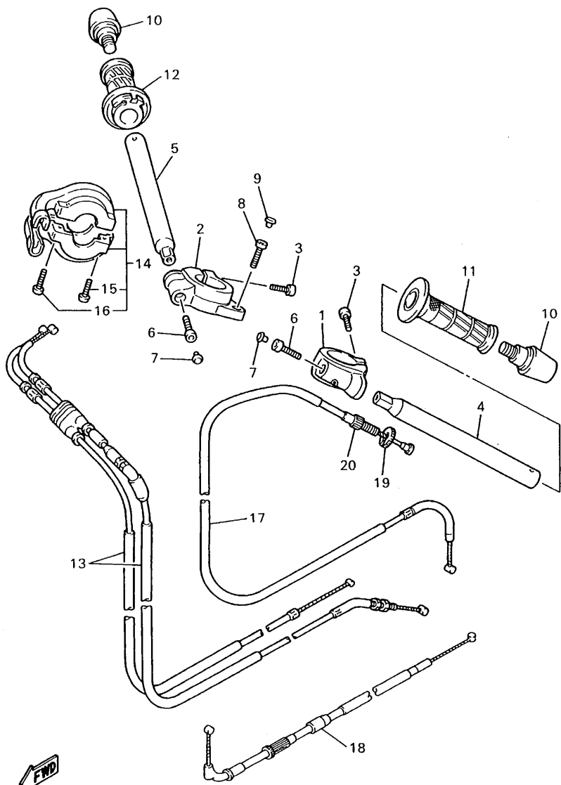
FIG. 33 MANUBRIO. CABLE
