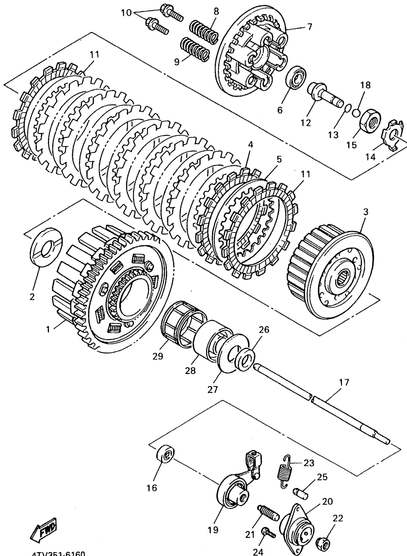
FIG. 16 EMBRAGUE
